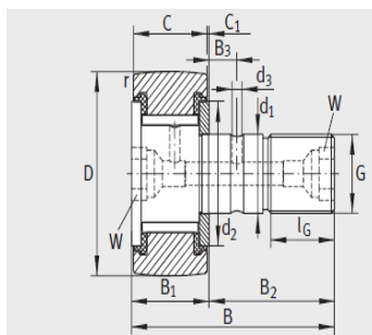
KRV...-PP (优化的 INA 轮廓形状)
