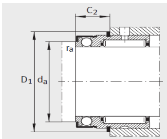
安装尺寸 外圈带卡环
