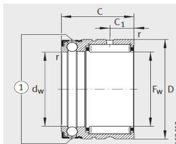
NX ① 润滑油孔
