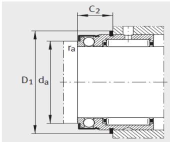
安装尺寸 外圈带卡环
