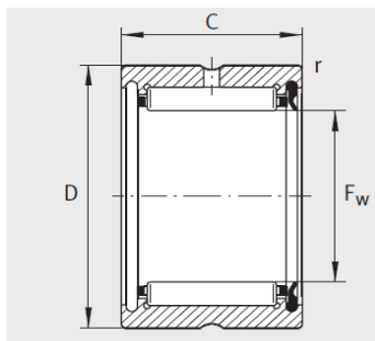
RNA4905-RSR
