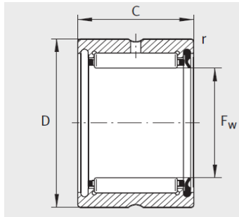
RNA4903-RSR
