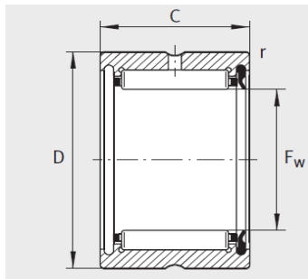
RNA4902-RSR
