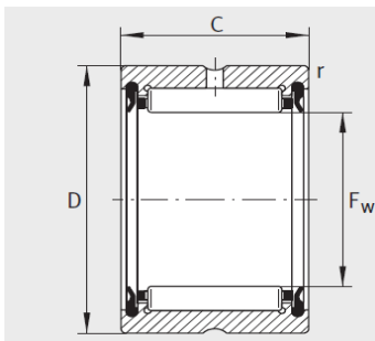
RNA4902-2RSR
