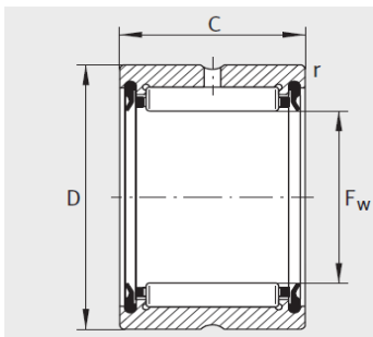
RNA4910-2RSR
